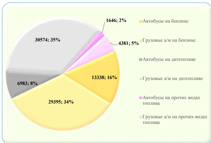
17. Состав парка дорожных механических транспортных средств в разбивке по видам используемого топлива в 2012 г.
