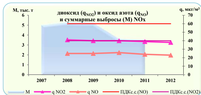
Рисунок 10 - Среднегодовые концентрации диоксида (qNO 2 ) и оксида азота (qNO) и суммарные выбросы (M) NO x (в пересчете на NO 2 )
